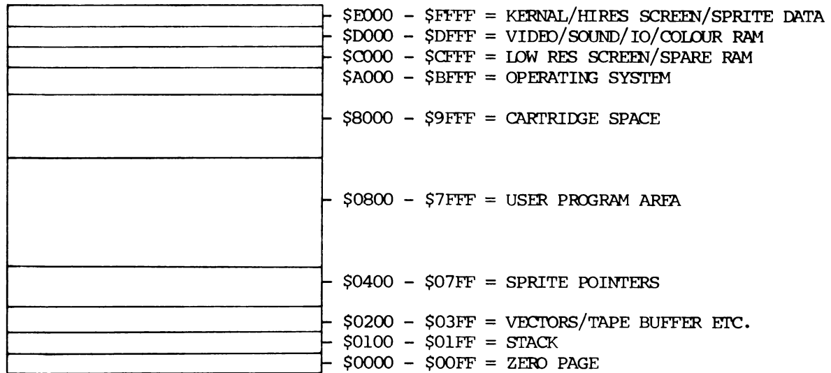
FIGURA 8-2 CONFIGURAZIONE DI MEMORIA DOPO MEM
