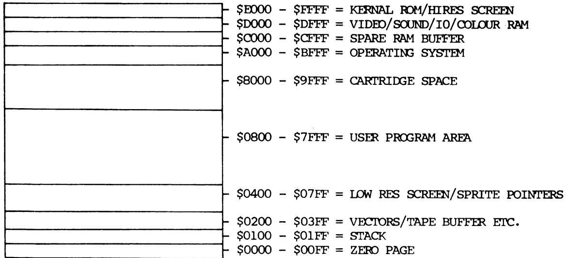
FIGURA 8-1 CONFIGURAZIONE DI MEMORIA PRIMA MEM
